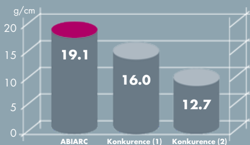
Hmotnost odstraněného kovu v závislosti na délce spotřebované elektrody
